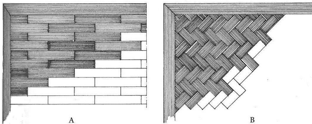
Afb. 1: Parketvloeren samengesteld uit kleine massieve stroken in lopend verband (A) en visgraatverband (B).
